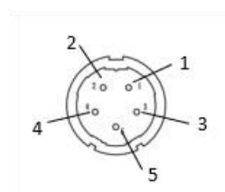
Connecteur 5 broches
